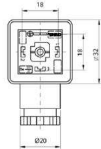
DIN 43650-A
