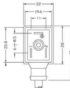
DIN 43650-B
